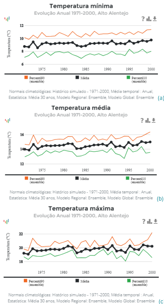
Figura 32. Evolução da temperatura mínima (a), média (b) e máxima (c) para a Região do Alto Alentejo, para o período 1971-2000
