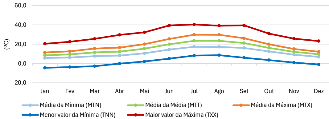
Figura 30. Temperatura do ar segundo as normais climatológicas para o período 1971-2000 | Estação Meteorológica de Portalegre
