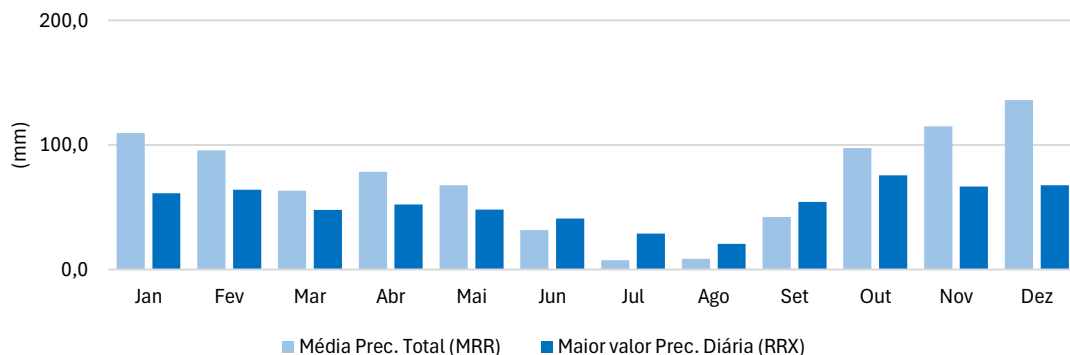
Figura 31. Precipitação segundo as normais climatológicas para o período 1971-2000 | Estação Meteorológica de Portalegre
